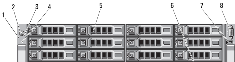
图 1-2. 前面板部件和指示灯（具有 12 个硬盘驱动器的系统）
