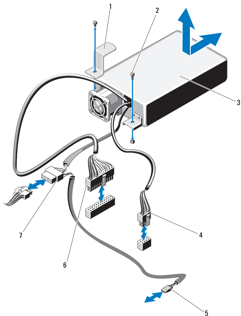
图 3-18. 卸下和安装非冗余电源设备
