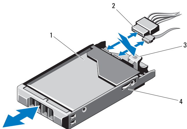
图 3-10. 卸下和安装已连接电缆的硬盘驱动器
