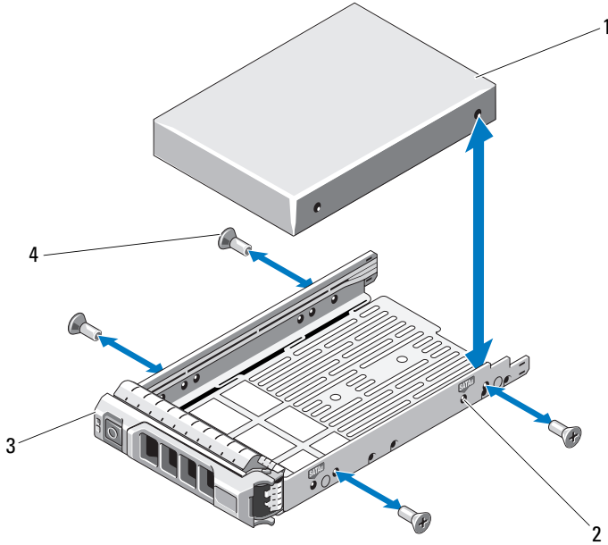
图 3-9. 将热交换硬盘驱动器安装到驱动器托盘中
