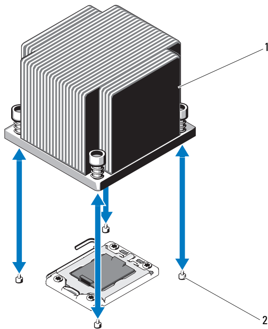
图 3-26. 安装和卸下散热器
