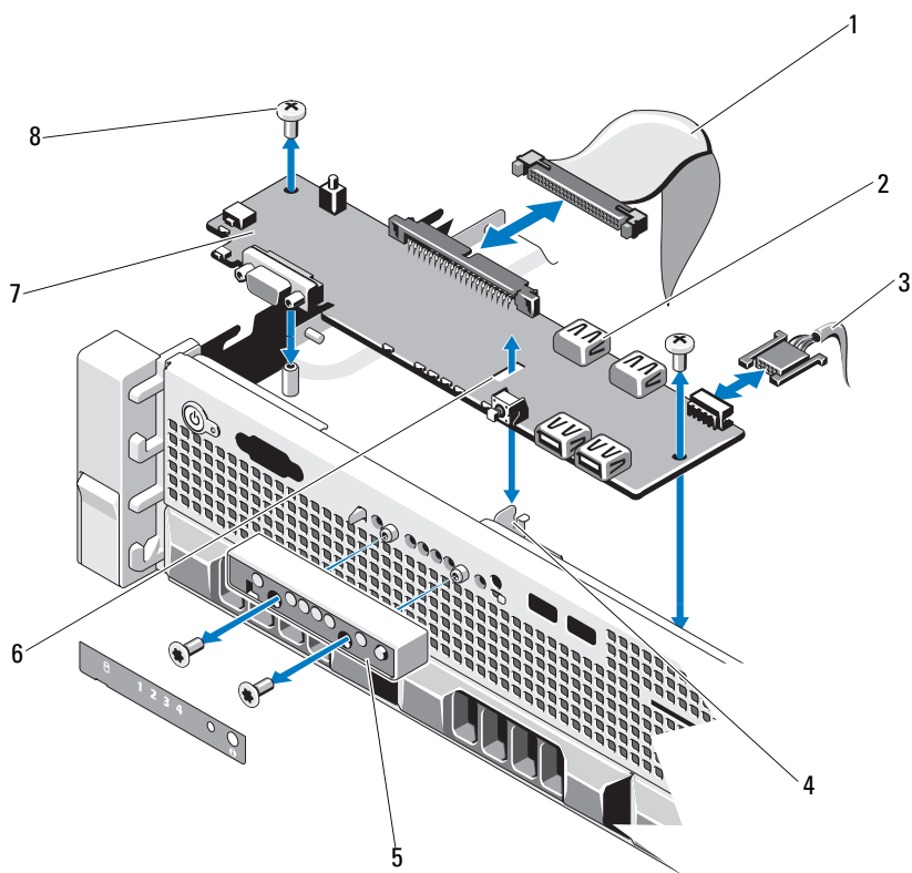
图 3-30. 卸下和安装控制面板—LED（具有 4 个硬盘驱动器的系统）
