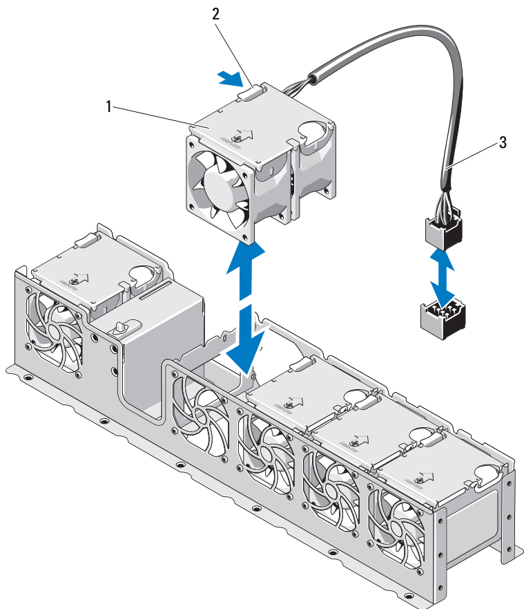
图 3-16. 卸下和装回风扇（具有 12 个硬盘驱动器的系统）
