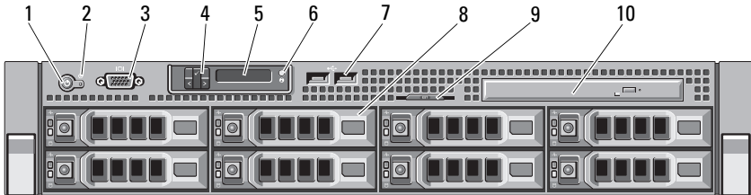
图 1-1. 前面板部件和指示灯（具有 8 个硬盘驱动器的系统）
