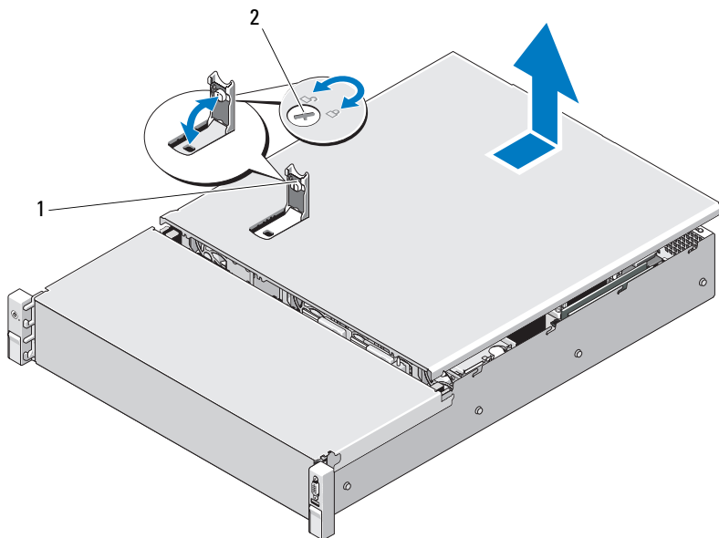
图 3-5. 卸下和装回系统护盖（具有 12 个硬盘驱动器的系统）
