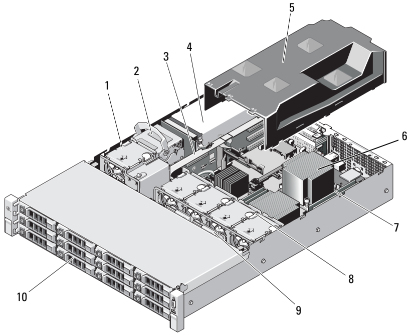
图 3-2. 系统内部组件（具有 12 个硬盘驱动器的系统）
