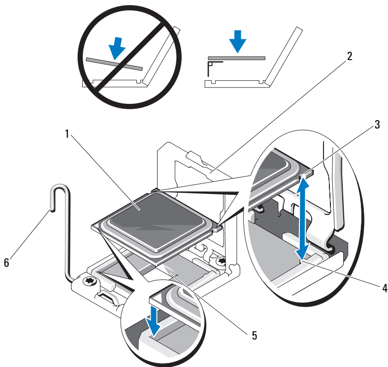
图 3-27. 安装和卸下处理器
