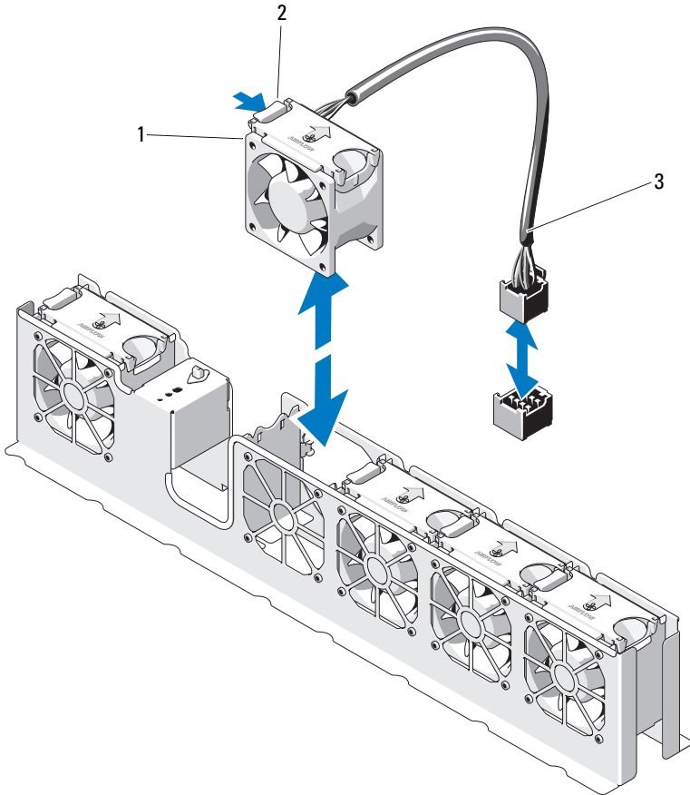
图 3-15. 卸下和装回风扇（具有 8 个硬盘驱动器的系统）
