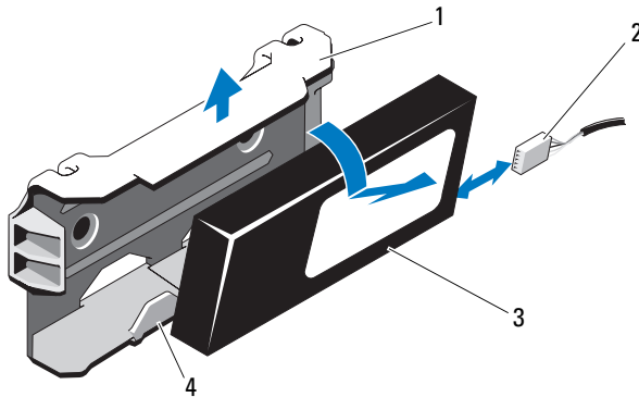
图 3-29. 卸下和安装 RAID 电池
