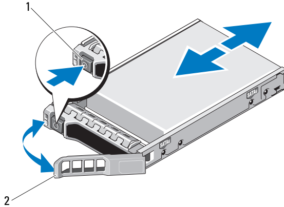
图 3-8. 卸下或安装热交换硬盘驱动器
