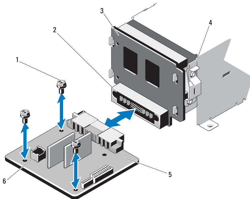
图 3-36. 卸下和装回配电板（具有 12 个硬盘驱动器的系统）
