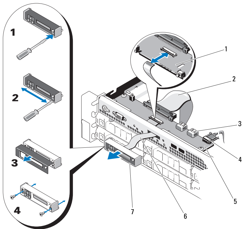
图 3-32. 卸下和安装控制面板 — LCD
