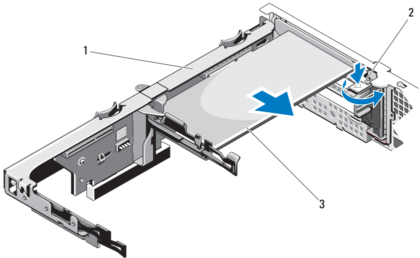
图 3-20. 安装或卸下扩充卡
