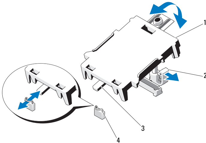
图 3-23. 安装或卸下 iDRAC6 Express 卡
