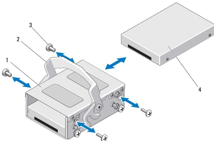
图 3-13. 在内部硬盘驱动器托架上安装内部硬盘驱动器
