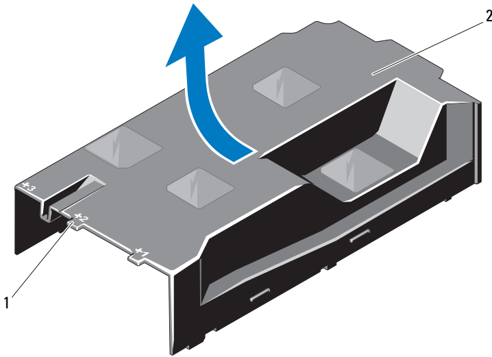
图 3-6. 安装和卸除冷却导流罩
