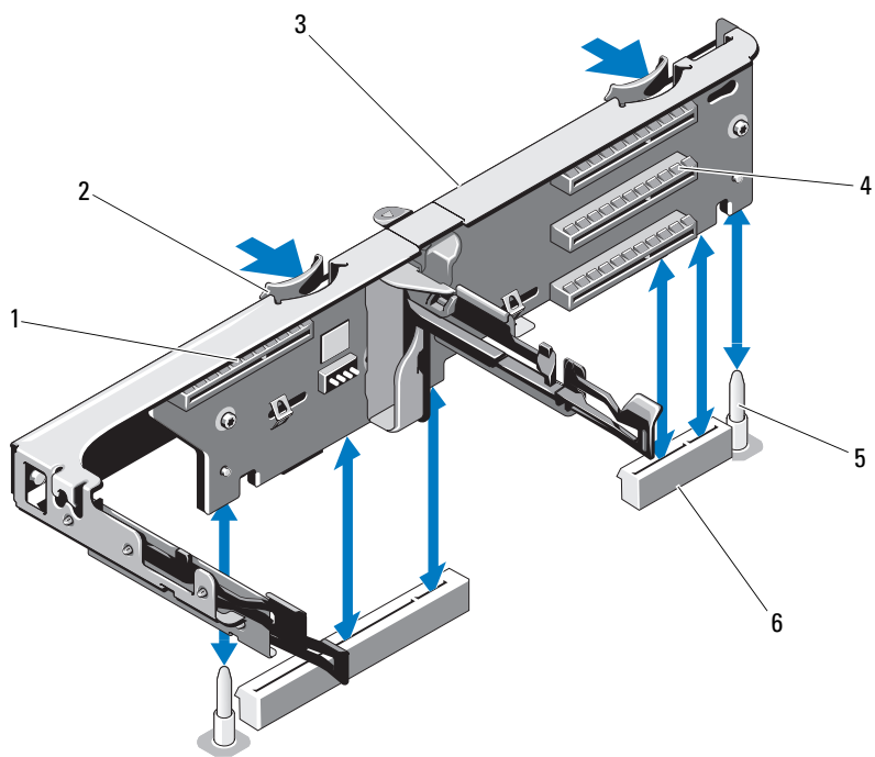
图 3-21. 安装或卸下扩充卡提升板
