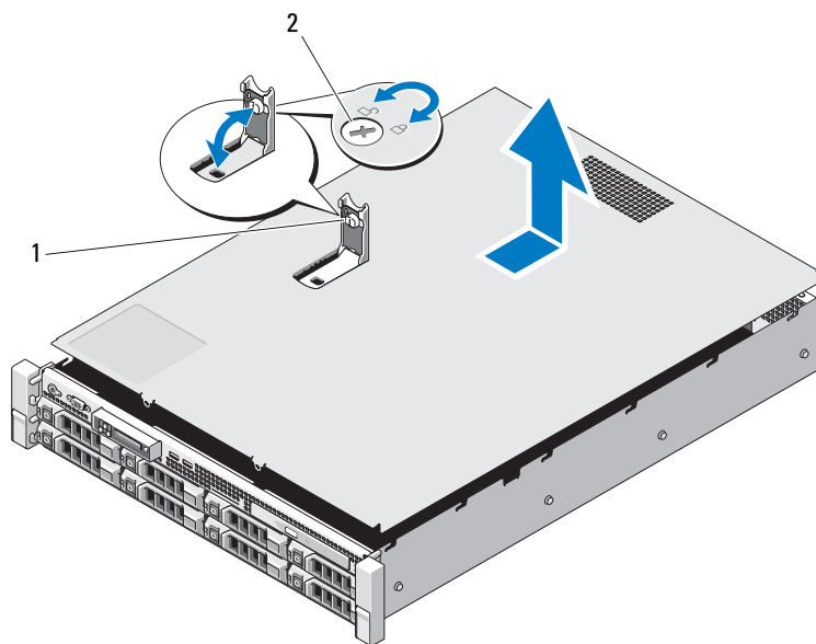
图 3-4. 卸下和装回系统护盖（具有 8 个硬盘驱动器的系统）
