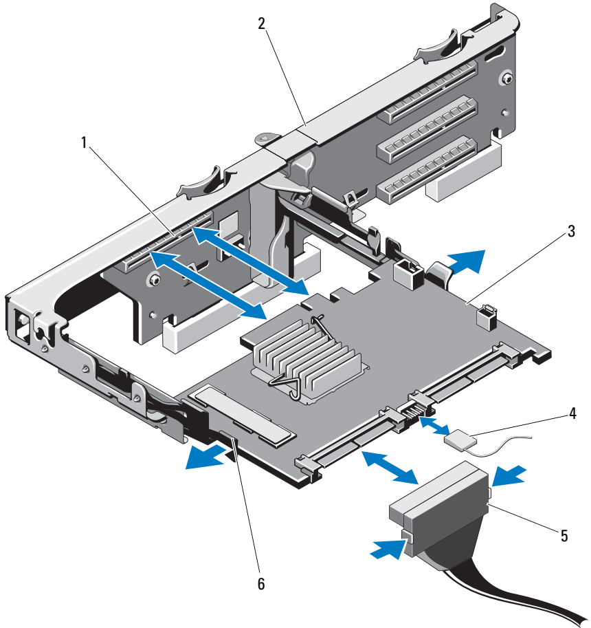
图 3-22. 安装和卸下存储控制器卡
