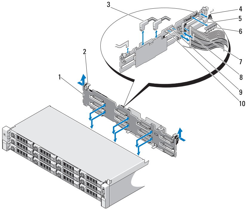
图 3-34. 卸下和安装 SAS 背板（具有 12 个硬盘驱动器的系统）
