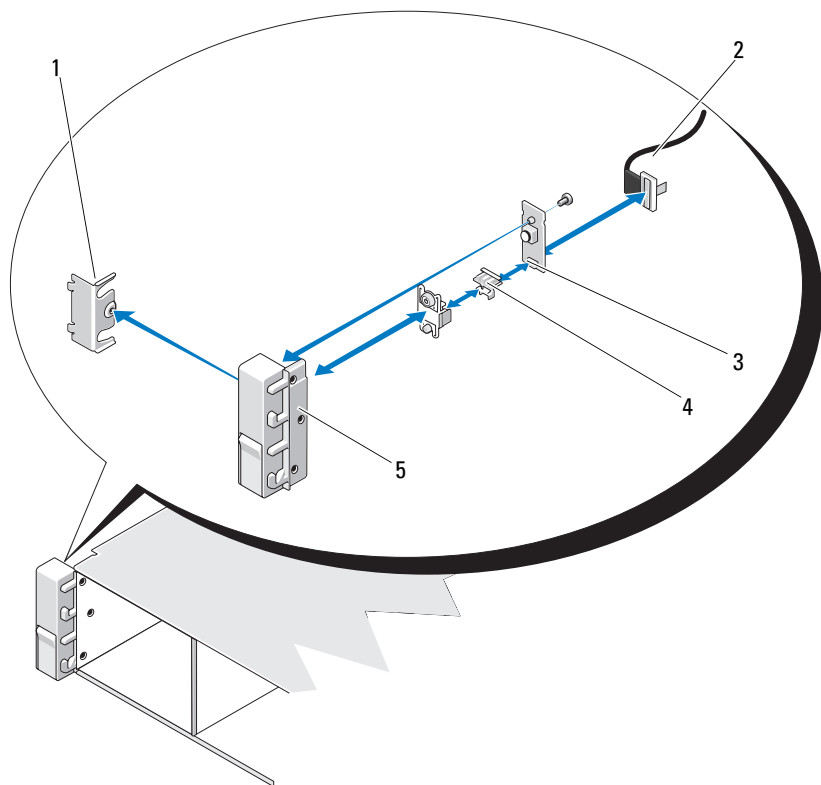
图 3-31. 卸下和安装控制面板—LED（具有 12 个硬盘驱动器的系统）
