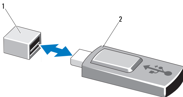
图 3-25. 卸下或安装 USB 存储钥匙
