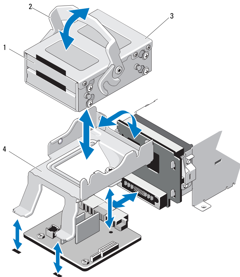
图 3-12. 安装和卸下内部硬盘驱动器托架
