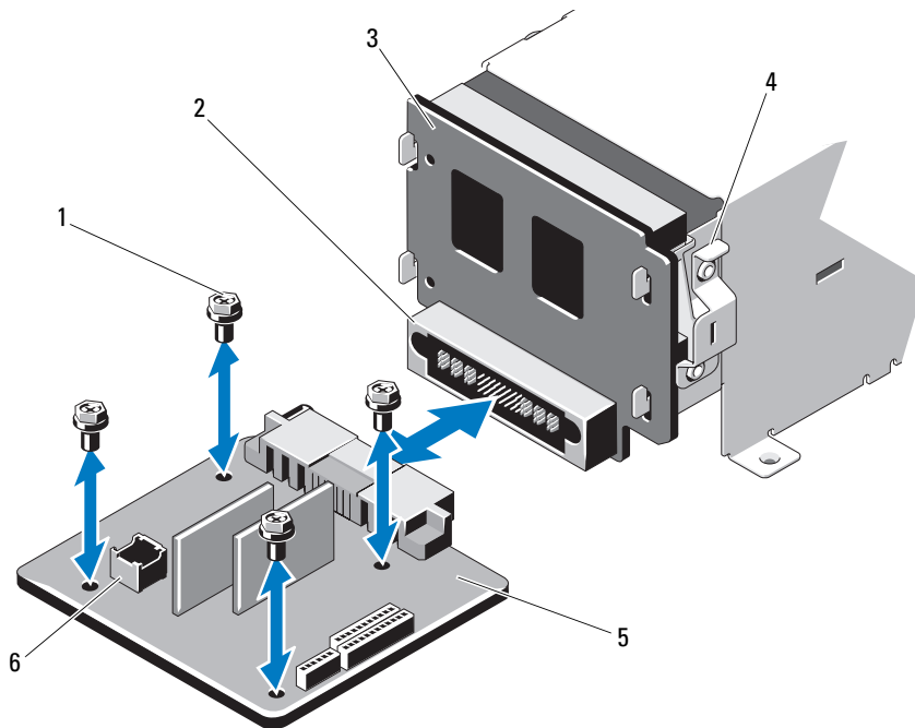
图 3-35. 卸下和安装配电板（具有 8 个硬盘驱动器的系统）
