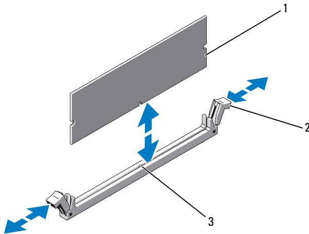
图 3-19. 安装和卸下内存模块
