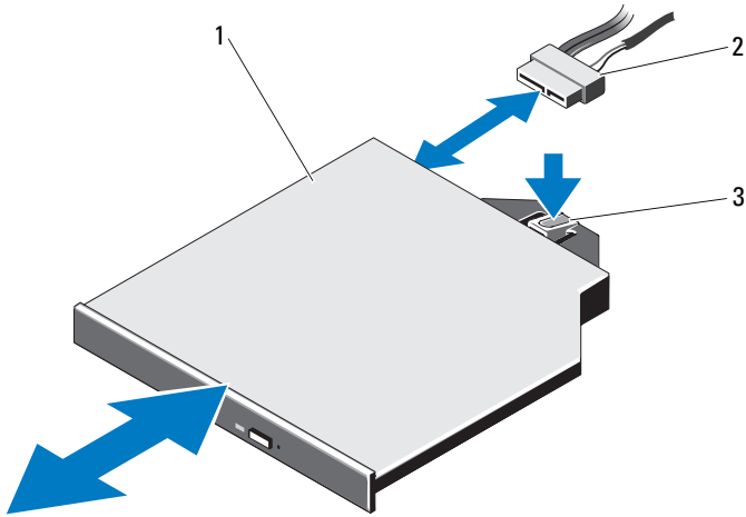
图 3-14. 卸下光盘驱动器
