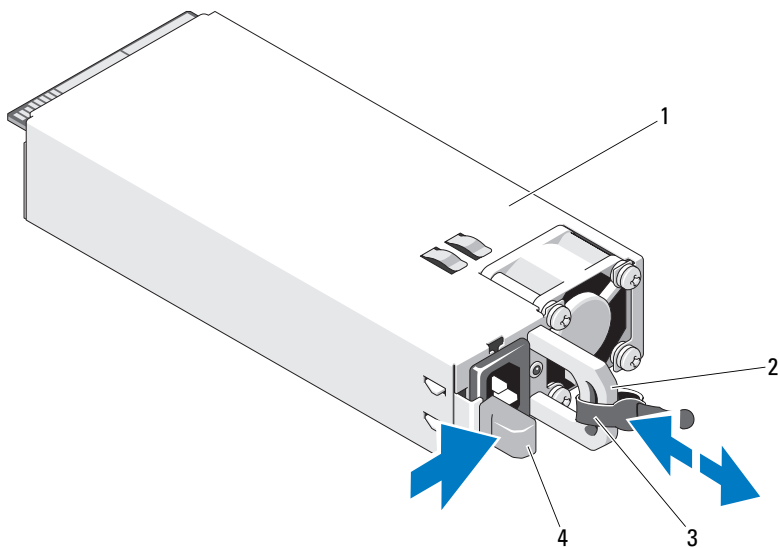
图 3-17. 卸下和安装冗余电源设备
