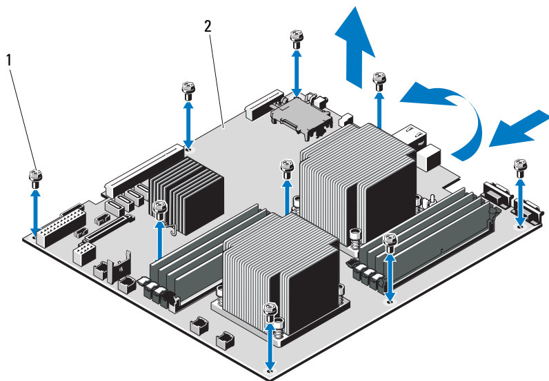
图 3-37. 卸下和安装系统板
