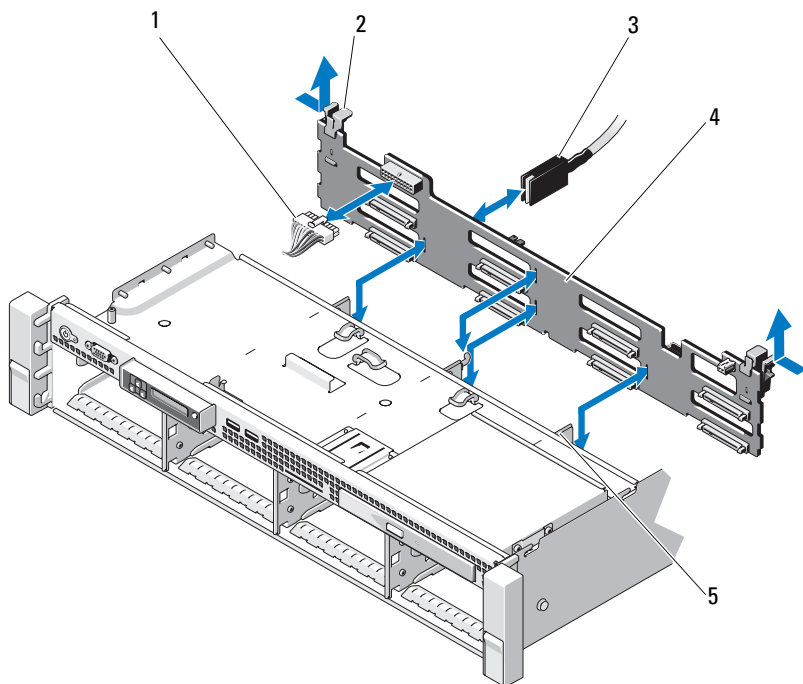
图 3-33. 卸下和安装 SAS 背板（具有 8 个硬盘驱动器的系统）
