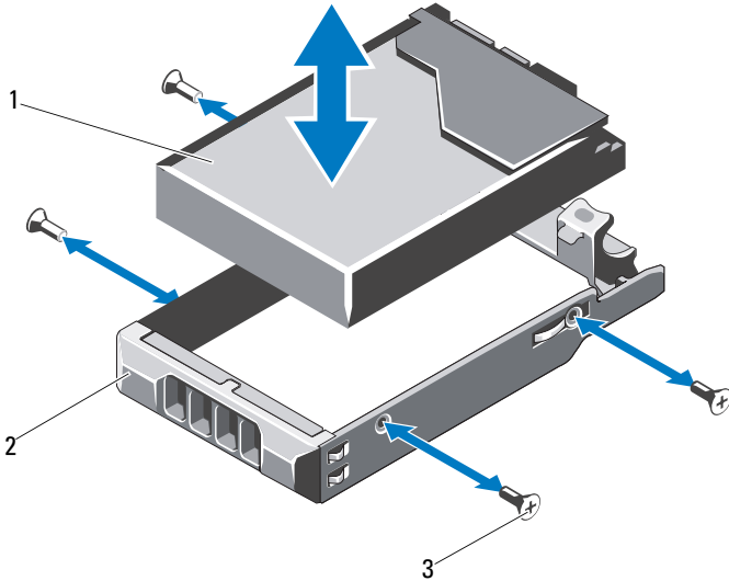
图 3-11. 将已连接电缆的硬盘驱动器安装到硬盘驱动器托盘中
