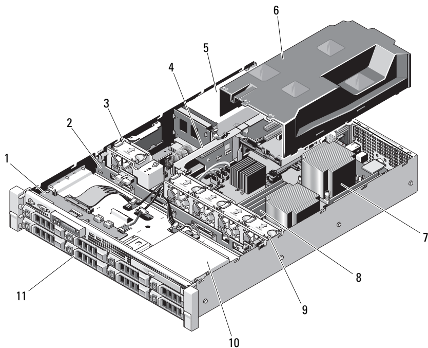
图 3-1. 系统内部组件（具有 8 个硬盘驱动器的系统）
